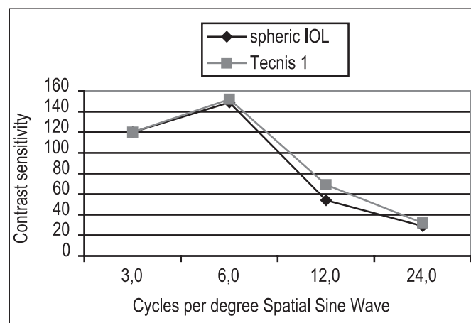
Graf 1. Porovnanie citlivosti na kontrast za fotopických podmienok
