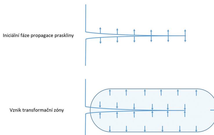
Obr. 1 Transformační zóna zapříčiní sevření praskliny
