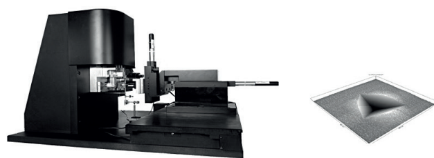
Obr. 5 Nanoindenter
