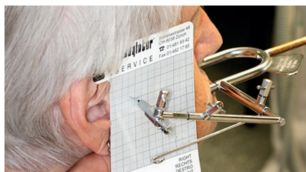
Obr. 7 Grafická registrace úhlu podélného sklonu kloubní dráhy na registrační papír s milimetrovým síťovým měřítkem
