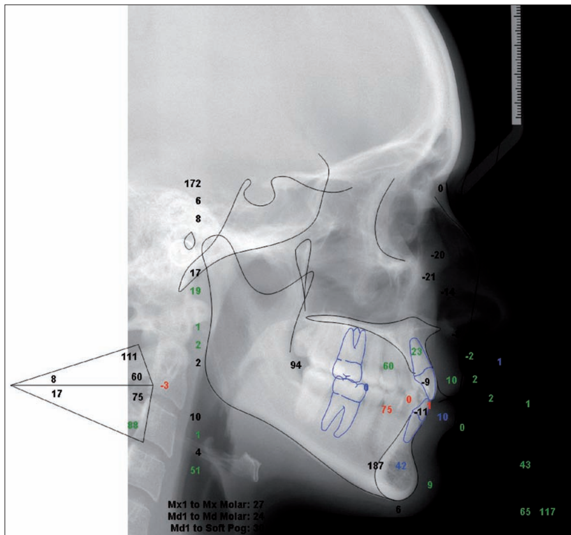
Obr. 1 Ukázka McLaughlinovy kefalometrické analýzy – program Dolphin Imaging
