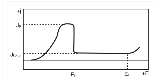
Graf 6. Polarizační křivka kovu přecházejícího do pasivního stavu: E_p – pasivační potenciál, E_t – transpasivační potenciál, j_p – kritická pasivační proudová hustota, j_{kor,p} – korozní proudová hustota v pasivním stavu.
