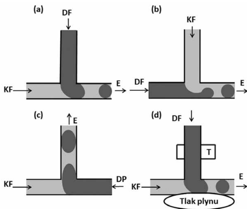
Obr. 2. Uspořádání typu T (přepřevzato dle 16) ): a – standardní T uspořádání, b – T uspořádání se vstříkovaním disperzní fáze přes hlavní kanál, c – T uspořádání s „head-on“ geometrií, d – aktivní T geometrie s řízenou pohyblivou konstrukcí stěn, zde zvýšením tlaku vzduchu/plynu v přiléhající struktuře DF – dispergovaná fáze, KF – kontinuální fáze, E – emulze
