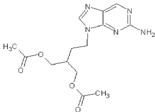
Obr. 3. Struktura famcikloviru
