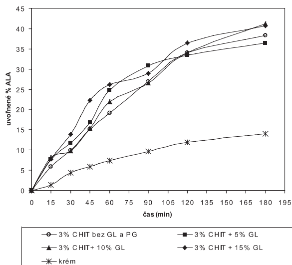
Obr. 1. Liberačný profil ALA z 3% chitosanových hydrogélů bez a s obsahem GL v porovnaní s liberáciou ALA z krému
