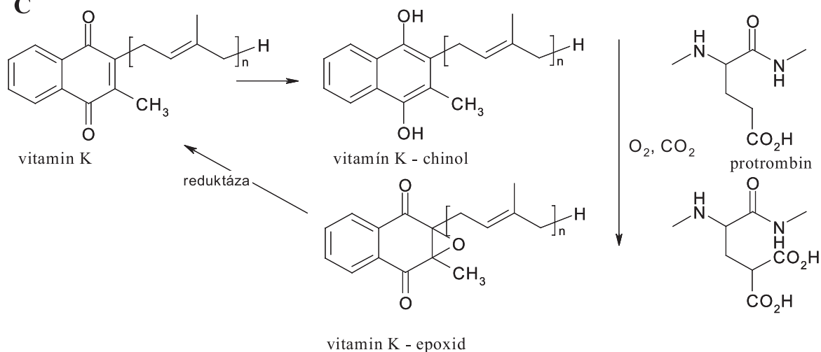
Obr. 2A) Struktura vitaminů K_1 a K_2 , B) vznik menachinonu z 1,4-dihydroxynafthoquinonové kyseliny, C) vitaminy skupiny K a krevní srážení, vztah vitaminů K k protrombinu
