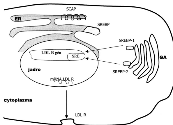
Obr. 3. Oplynenie expresie LDL receptora pomocou génovej transkripcie cez SREBP-SCAP cestu
