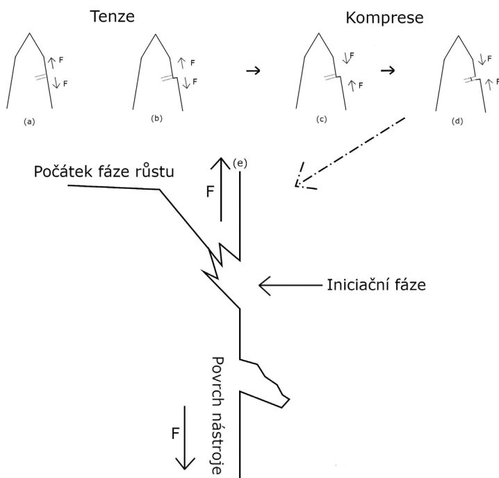
Obr. 3 Iniciační fáze fraktury na podkladě cyklické únavy, podélný řez nástrojem (a–d) Dislokace hmoty na povrchu nástroje v průběhu cyklu, formace perzistentních skluzových pásů; (e) Stav povrchu po opakované cyklické zátěži nástroje, přítomné skluzové pásy a mikroprasklina, která přechází do fáze růstu; ↑F, ↓F Směr působící aplikované síly
