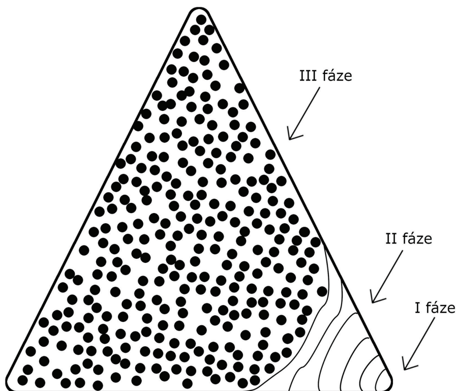
Obr. 2 Schéma plochy lomu endodontického nástroje I. fáze – vznik praskliny; II. fáze – postupný růst praskliny, přítomny charakteristické pruhy; III. fáze – terminální fraktura, chaotický povrch lomné plochy
