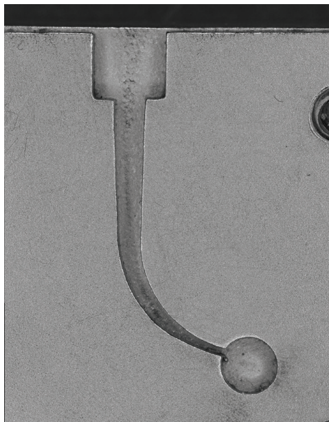
Obr. 4 Individuální kanál z nerezové oceli pro testování cyklické únavy
