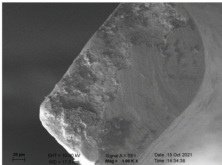
Obr. 1 Lomná plocha endodontického nástroje po testu cyklické únavy při zvětšení 1000× ve skenovacím elektronovém mikroskopu
