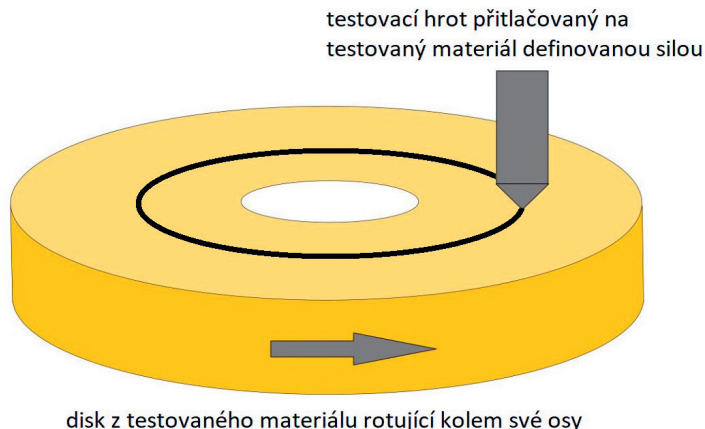
Obr. 2 Princip Pin on disc metody měření opotřebení materiálů
