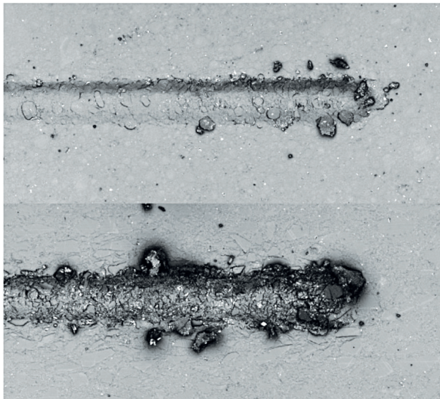
Obr. 6 CLSM obraz vrypů flow kompozitního (nahore) a pastovitěho nanohybridního kompozitního materiálu (dole)
