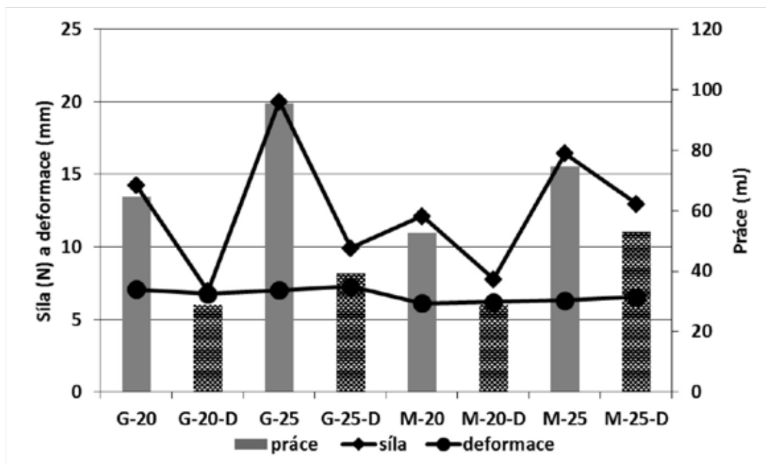
Obr. 3. Mechanické vlastnosti filmů v suchém stavu
