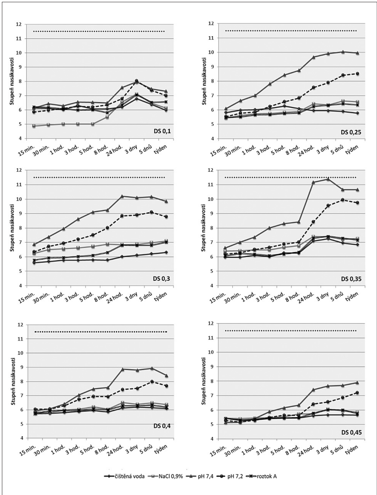
Obr. 1. Nasákavost kyselý formy CMC s DS od 0,1 do 0,45 v různých médiích
