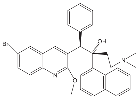
Obr. 4. Struktura antituberkulotika TMC207
