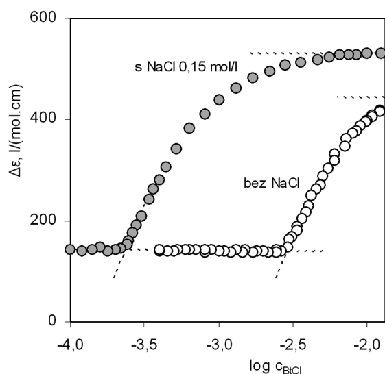
Obr. 4. Závislost rozdílu molárních absorpčních koeficientů benzethonium chloridu změřených při dvou vlnových délkách ( \Delta\epsilon = \epsilon_2 - \epsilon_1 , \text{l}\cdot\text{mol}^{-1}\cdot\text{cm}^{-1} ) na logaritmu koncentrace BtCl (jednotky c_{\text{BtCl}} mol/l), v roztocích bez přídavku a s přídavkem NaCl 0,15 mol/l
