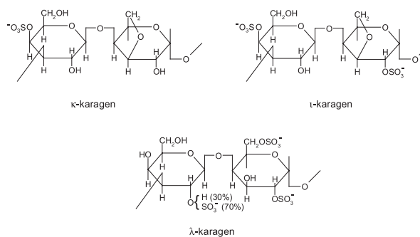
Obr. 4. Strukturální vzorec karagenů
