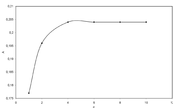
Obr. 2. Závislost absorbance chloroformového výtřepku iontového páru BEC-2,4-dinitrofenol na molárním přebytku 2,4-dinitrofenolu ( E ) při koncentraci tenzidu 1 \cdot 10^{-4} mol/l, pH=7,00 , \lambda_{max}=420 nm a t=30 min
