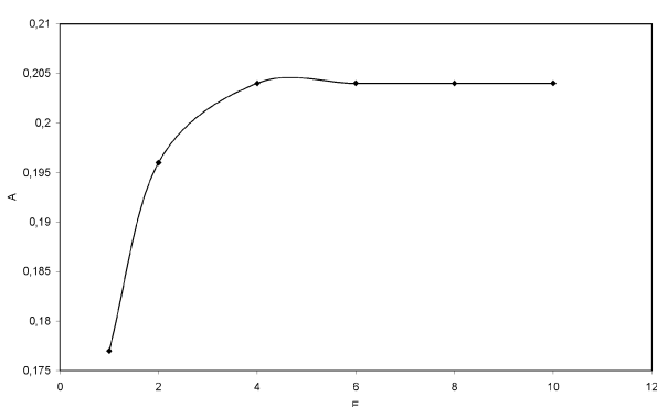
Obr. 2. Závislost absorpance chloroformového výtřepku iontového páru BEC-2,4-dinitrofenol na molárním přebytku 2,4-dinitrofenolu ( E ) při koncentraci tenzidu 1 \cdot 10^{-4} mol/l, pH=7,00 , \lambda_{max}=420 nm a t=30 min
